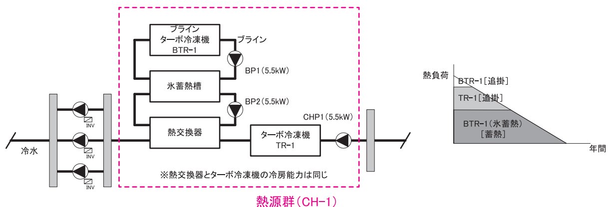
図 2-2-27 蓄熱システムを他熱源機器と直列に組み合わせた例
