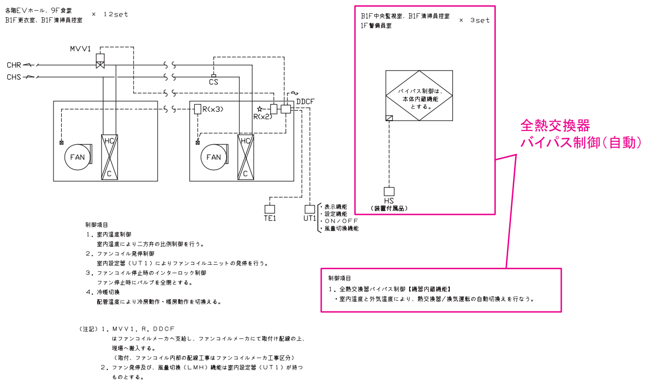
図 3-2-35 空調設備自動制御フロー図 (6) (図面 - 空 -23 : 全熱交換器部分を抜粋)
