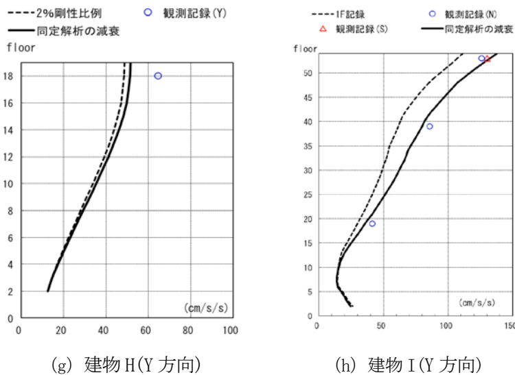
図 4.4-16 応答解析の加速度応答と観測記録(2/2)
