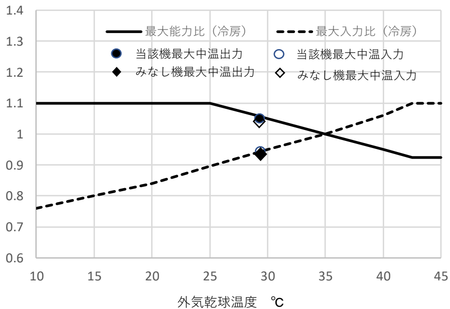
図3 中温条件最大能力時（冷房）における当該機の試験値、みなし機の試験値、及びビル用マルチエアコン（都市ガス式）最大能力比特性及び最大入力比特性（冷房）の比較
