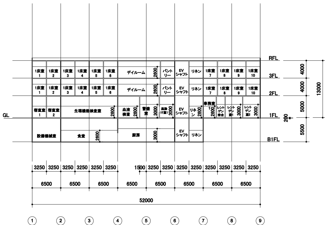
モデル建物（総合病院、5,000㎡） A-A' 断面図 1/300
