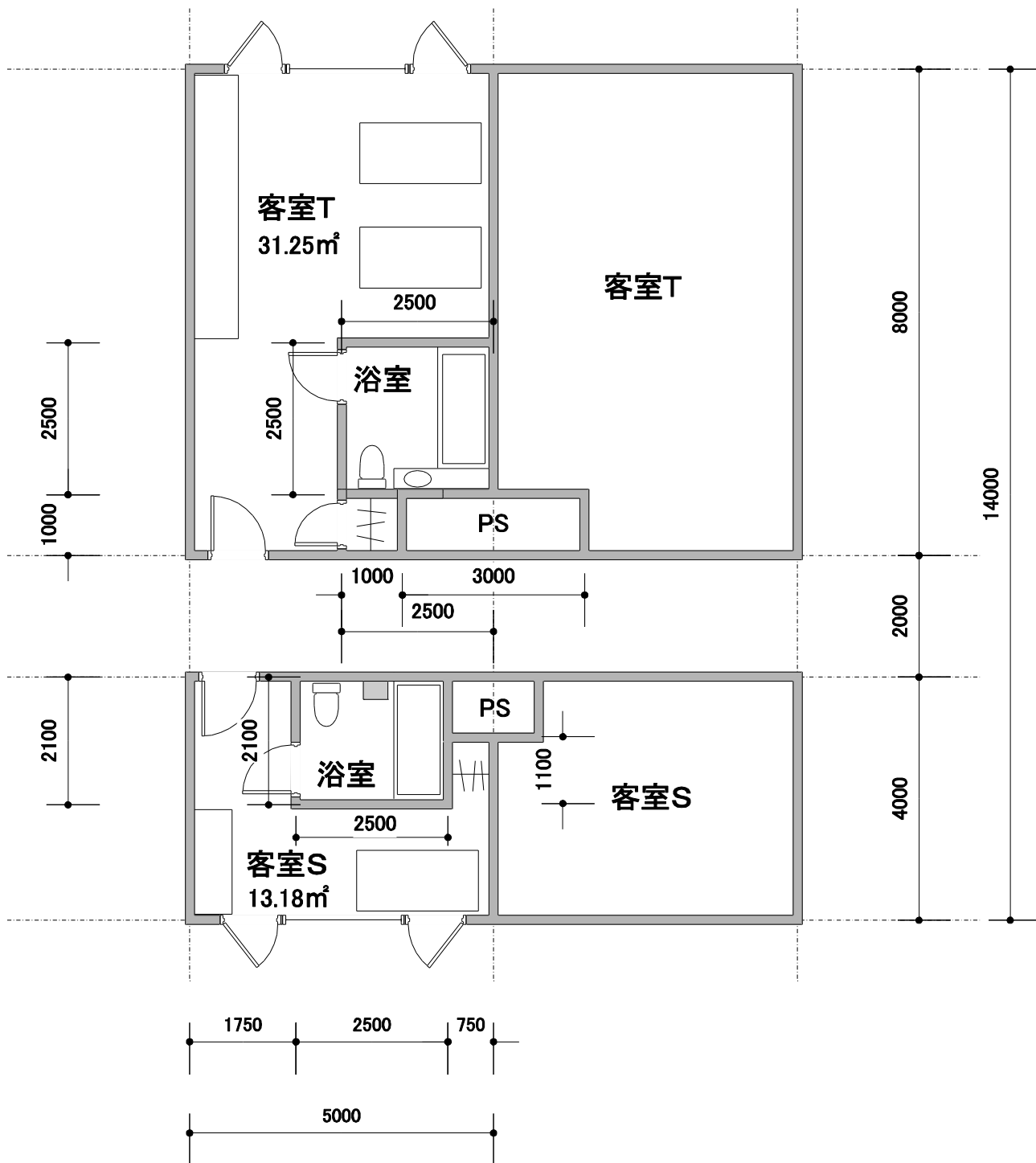
モデル建物（シティホテル、16,700m²） 客室基準平面図 1/100
