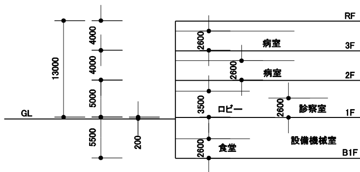
モデル建物（総合病院、5,000㎡） 階高及び天井高
