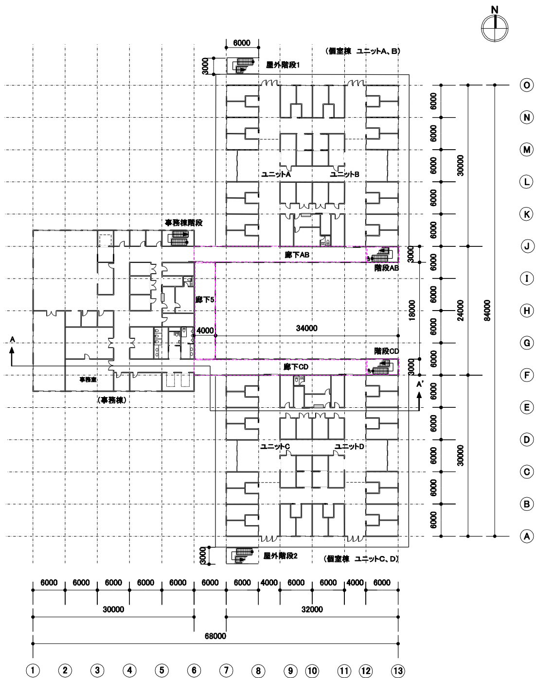
モデル建物（福祉施設、6,240㎡） 2階平面図 1/500
