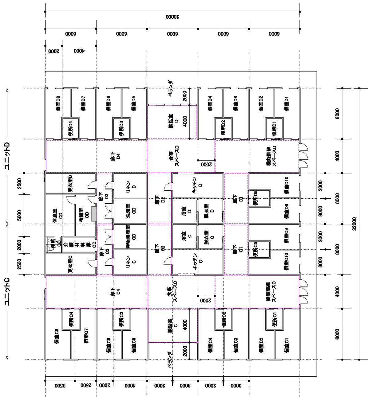
モデル建物（福祉施設、6,240㎡） ユニットC、D（個室棟）詳細図 1/200
