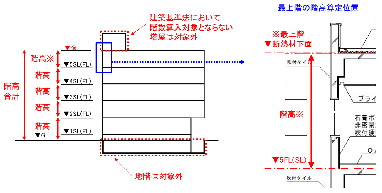
図 2-2-4 「各階の階高の合計」の算出方法 (最下階は GL から算出し、その他の階高はフロアレベル間で算出する場合)
