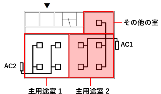
図 2-2 最大床面積の主用途室が複数ある場合-2
