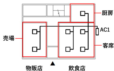
図2-7 1台の熱源機器（AC1）で異なる建築物用途を空調する場合
