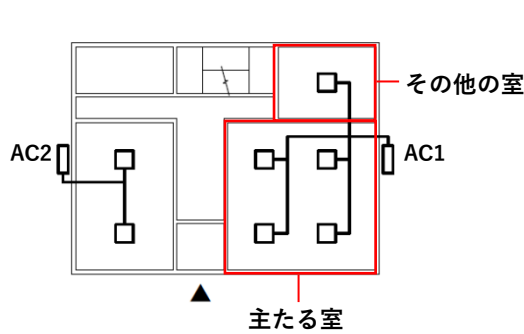
図2-4 最大熱源機器 (AC1) が主たる室以外の室を空調する場合
