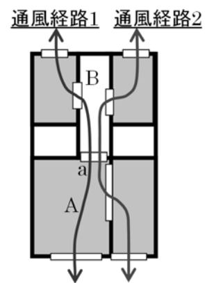
図 C.2 2本の通風経路が空間・開口部を重複して通過する例
