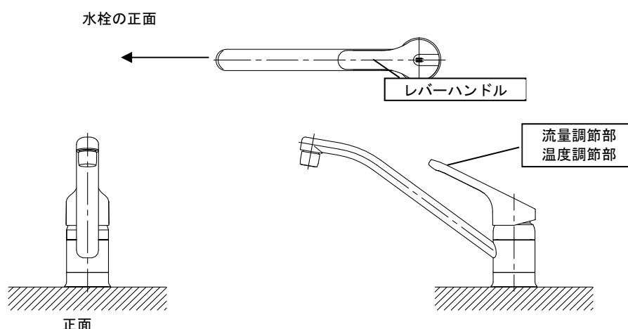
図 2 手元止水機構浴室－シャワー水栓の例
