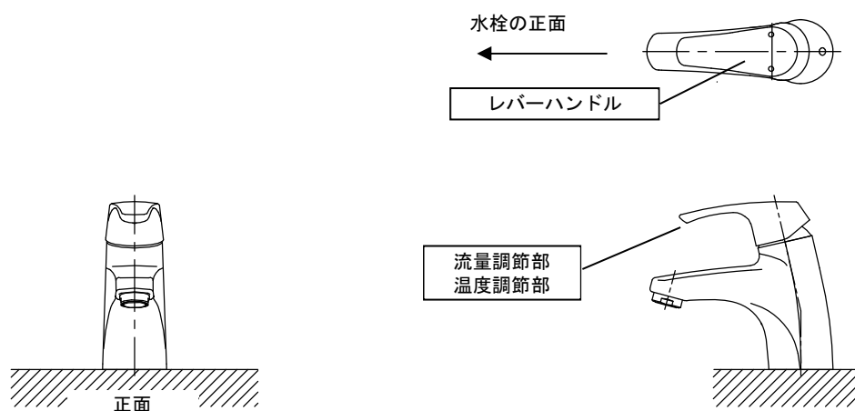
図 5 水優先吐水機構－台所水栓(レバーハンドルが水栓胴の左右側面に位置する場合)の例
