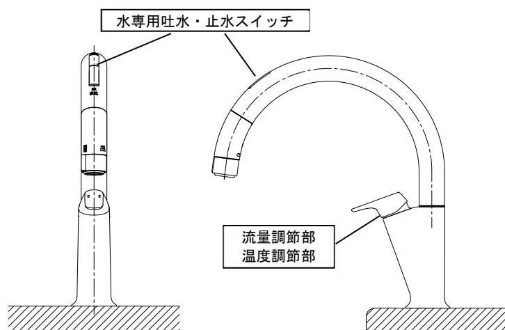
図 4 水優先吐水機構－台所水栓(水専用の吐水止水操作部)の例
