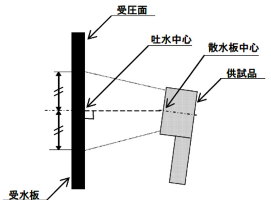
図 2 吐水角度概念図
