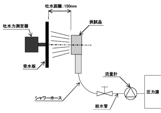
図 1 試験装置概要(イメージ図)
