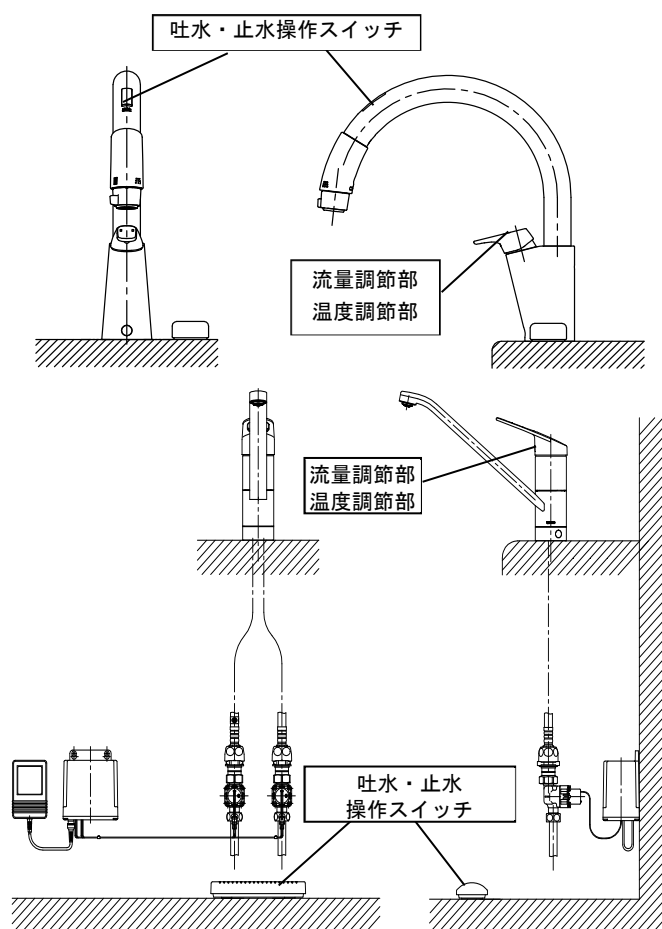
図 1 手元止水機構一台所水栓の例
