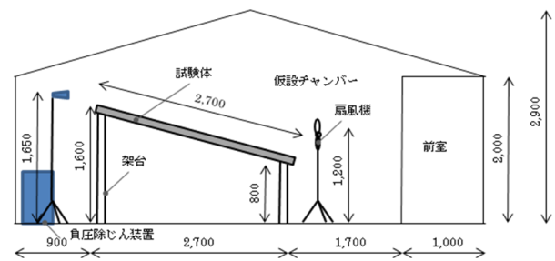
図2 仮設チャンバー及び測定状況の概要（単位：mm）
