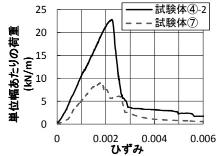
図 4 面内圧縮実験結果の例 （懐の長さの異なる天井の比較）
