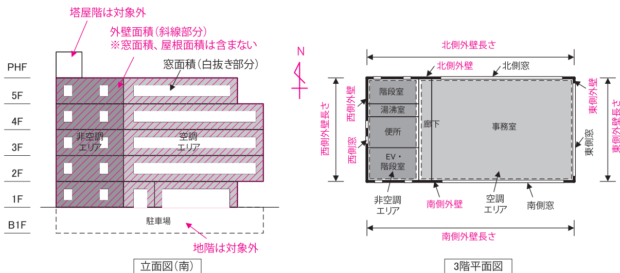
図 2.3.6 外壁面積の算出方法
