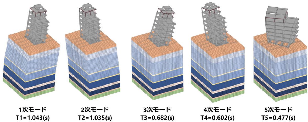
図 5.2-20 1～5 次モード図
