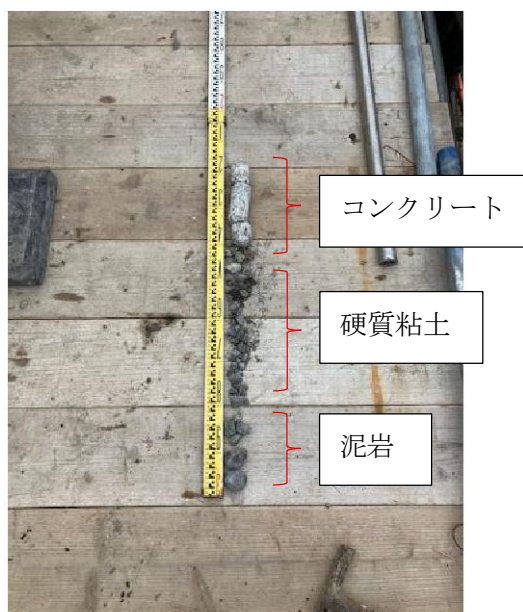
写真 3.4.1-2 杭先端シュウ以深から採取されたコンクリートコア
