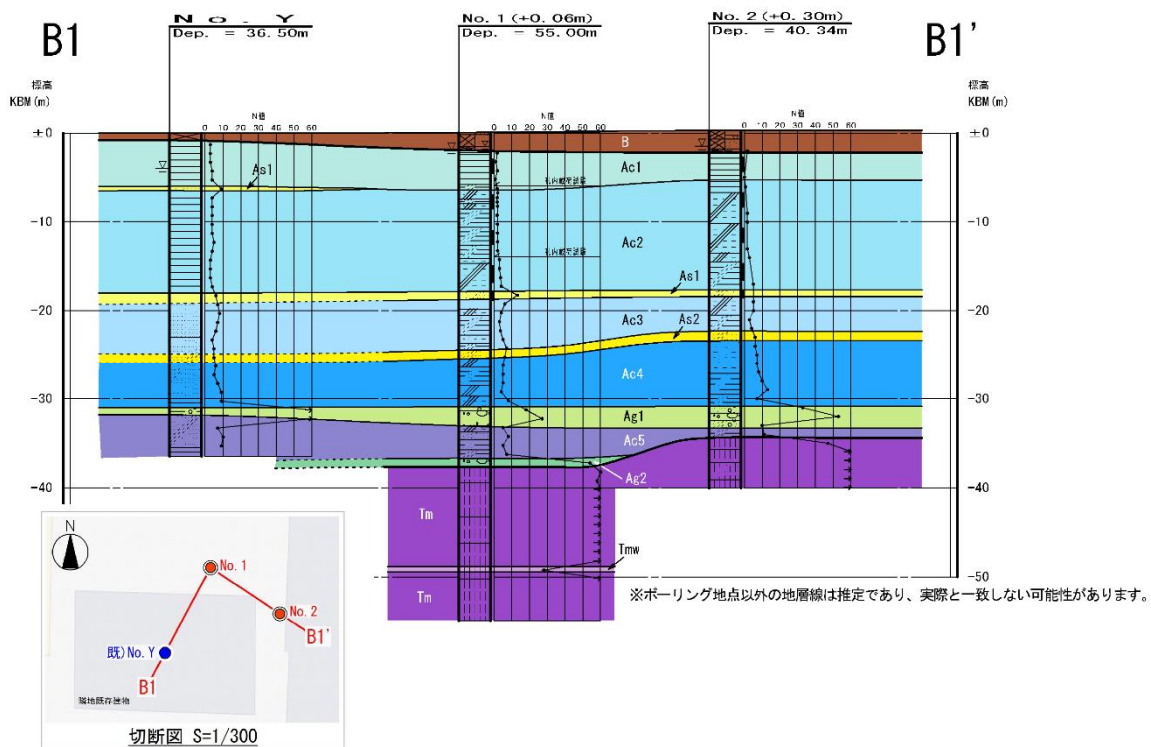
図 3.1.4-22 土質柱状図
