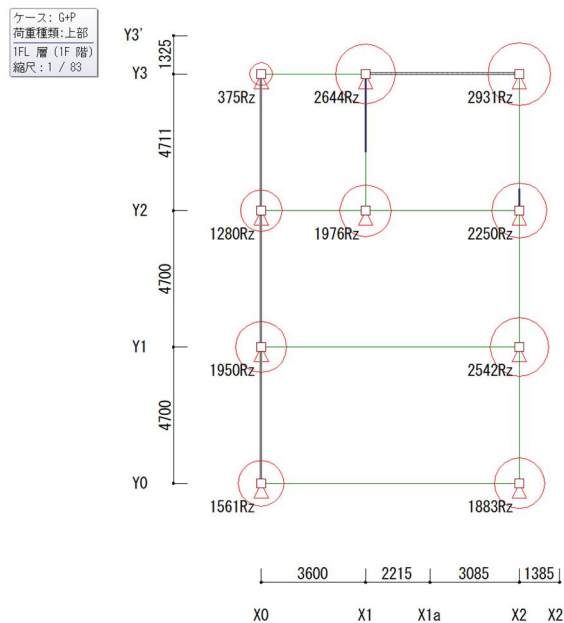
図 2.3.3-1 長期荷重時 支点反力
