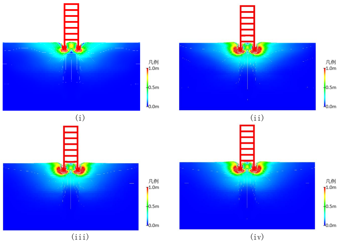
(b) A-2 全体変位 (Dxy)
