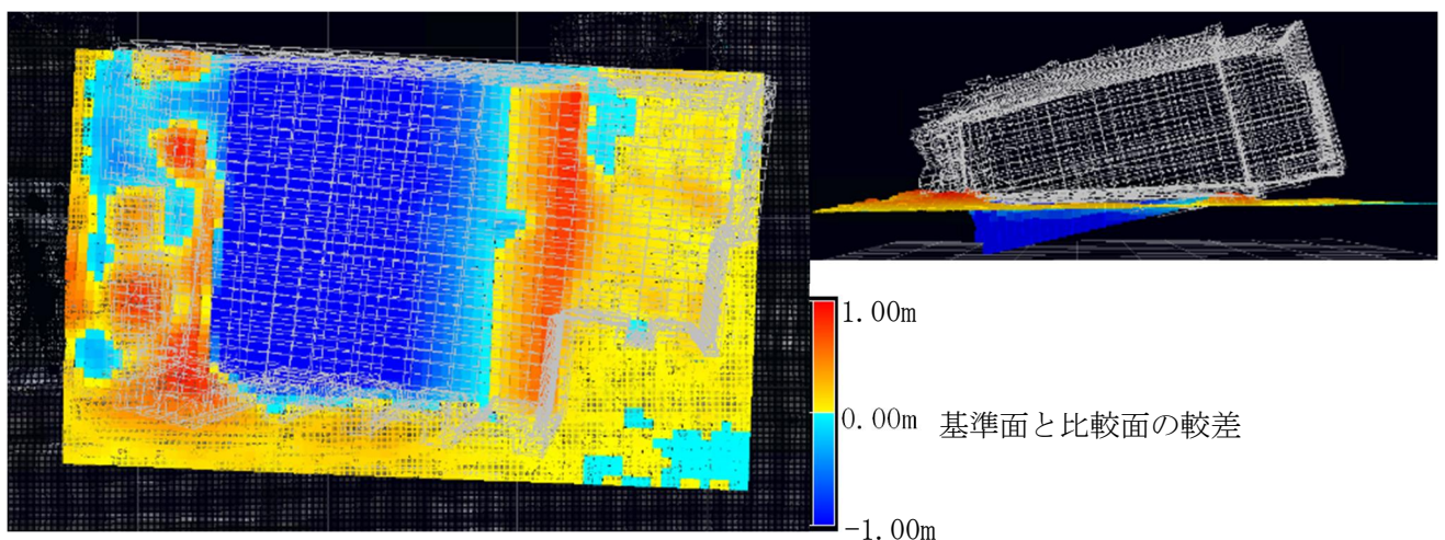
図 2.2.1-58 case-B の土量計算結果
