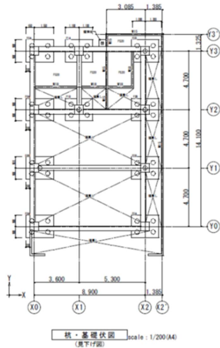
図 3.4.2-1 平面図および杭配置図
