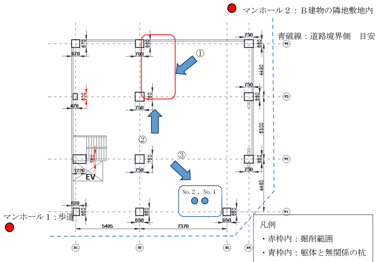
図 4.1.2-1 調査対象範囲と掘削範囲（目安）
