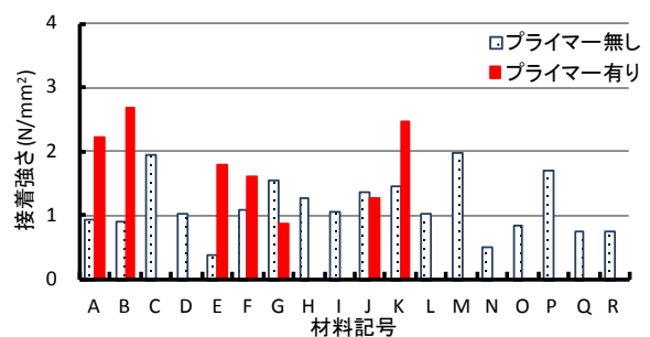
図-3.1.6 接着耐久性試験の結果
