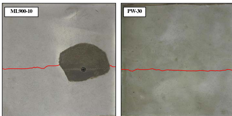
写真-3.2.1 耐火実験後の状況
