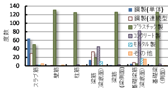
図-4.2.18 部材ごとのスペーサの種類
