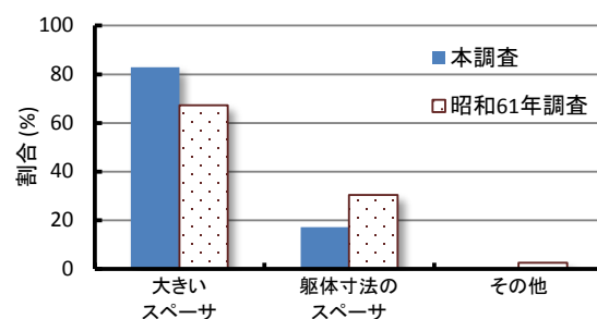
図-4.2.29 増打ちがある場合のスペーサの選定
