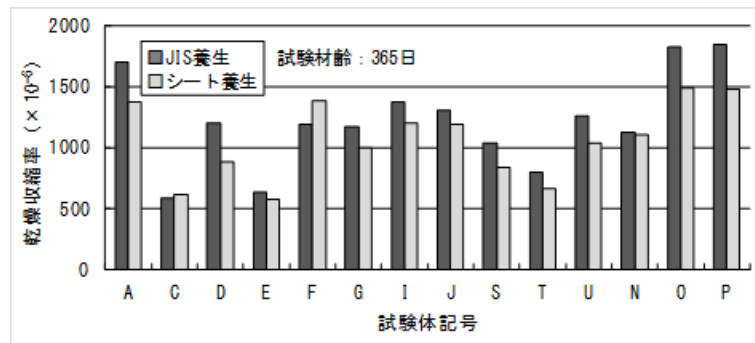
図-3.1.19 ポリマーセメントモルタル種類毎の乾燥収縮率(182日)
