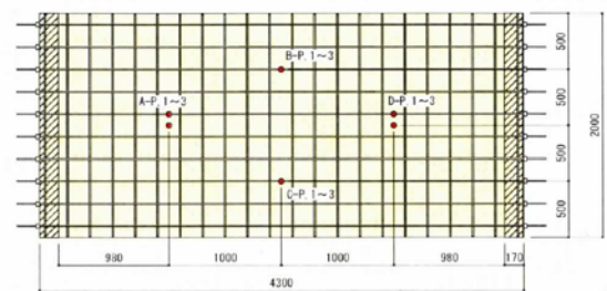
図 2 No.2 試験体の PCM 補修
