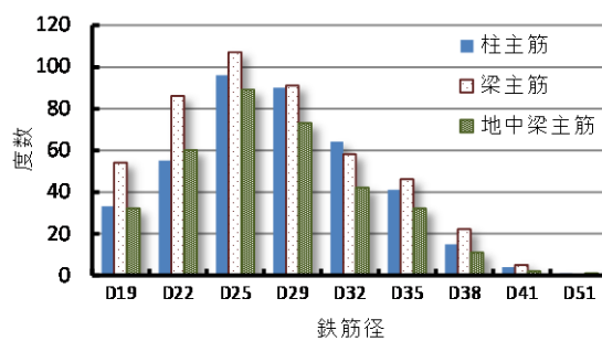
図-4.2.3 主筋の鉄筋径
