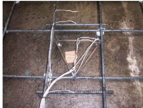
熱電対設置状況 1
