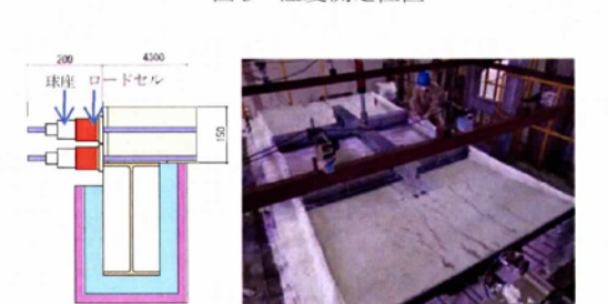
図 4 鉄筋端部張力測定 写真 3 実験状況
