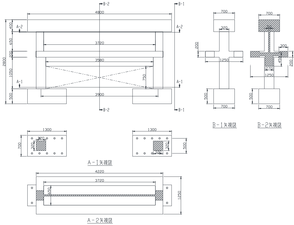
図 2 F2 試験体の外形図
