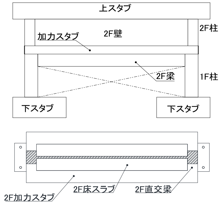
図 1 ピロティ架構試験体の各部名称定義
