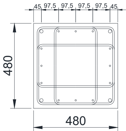
図2 ピロティ柱試験体断面図
