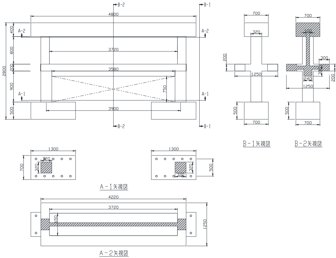
図 3 F3 試験体の外形図
