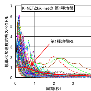
図 2 K-NET と kik-net で得られた第 1 種地盤(左)、第 2 種地盤(右)の規準化加速度応答スペクトル
