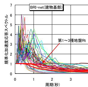
図 3 BRI-net の建物基部(左)、地盤(右)で得られた記録の規準化加速度応答スペクトル
