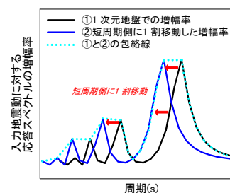
図 4 工学的基盤の傾斜を考慮した増幅係数の補正案
