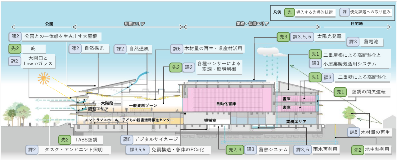
先導的な環境技術・取組イメージ断面図
